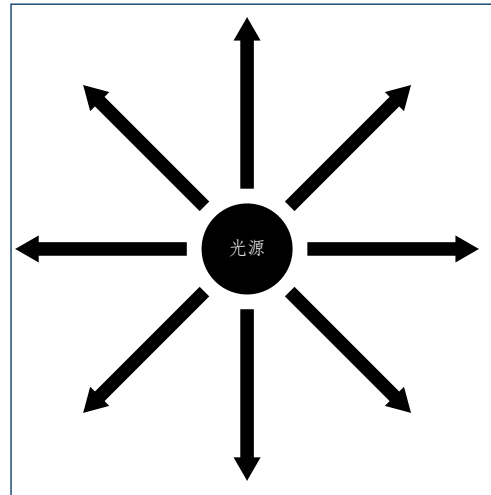
图14.光通量的演示。
