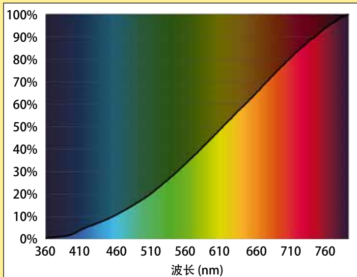
图8.白炽灯的光谱。
