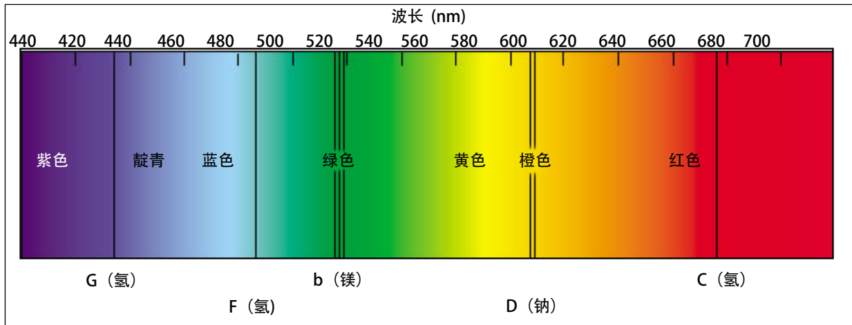
图4.可见光谱。
