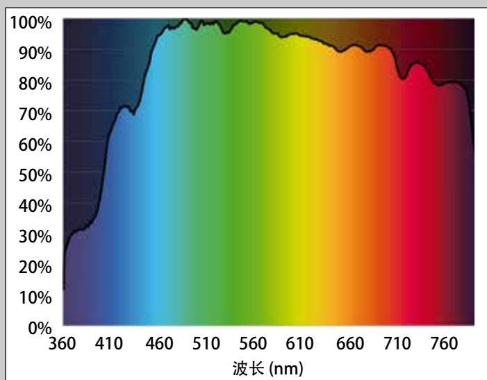
图7.中午的阳光光谱。
