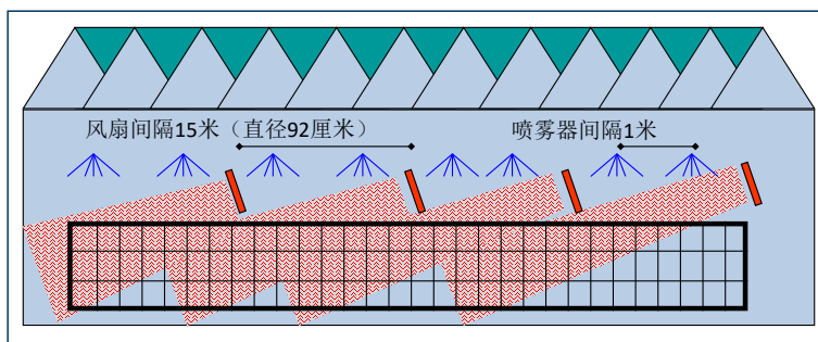
图5. 开放型鸡舍内安装搅拌风扇和喷雾器。
